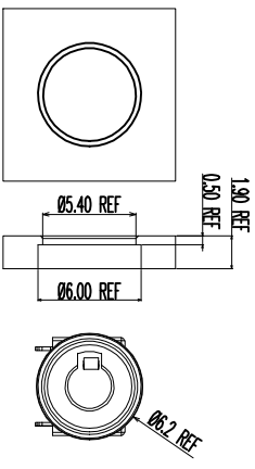
面接开孔参考尺寸
